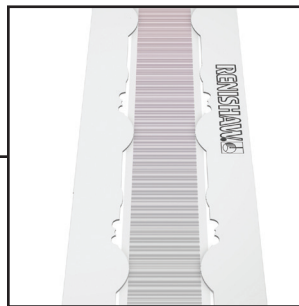
Riga a nastro RTLA50 e guida FASTRACK
