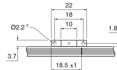
(고객 선택사항) 볼트형 레퍼런스 마크 선택기 및 리미트 마그넷
