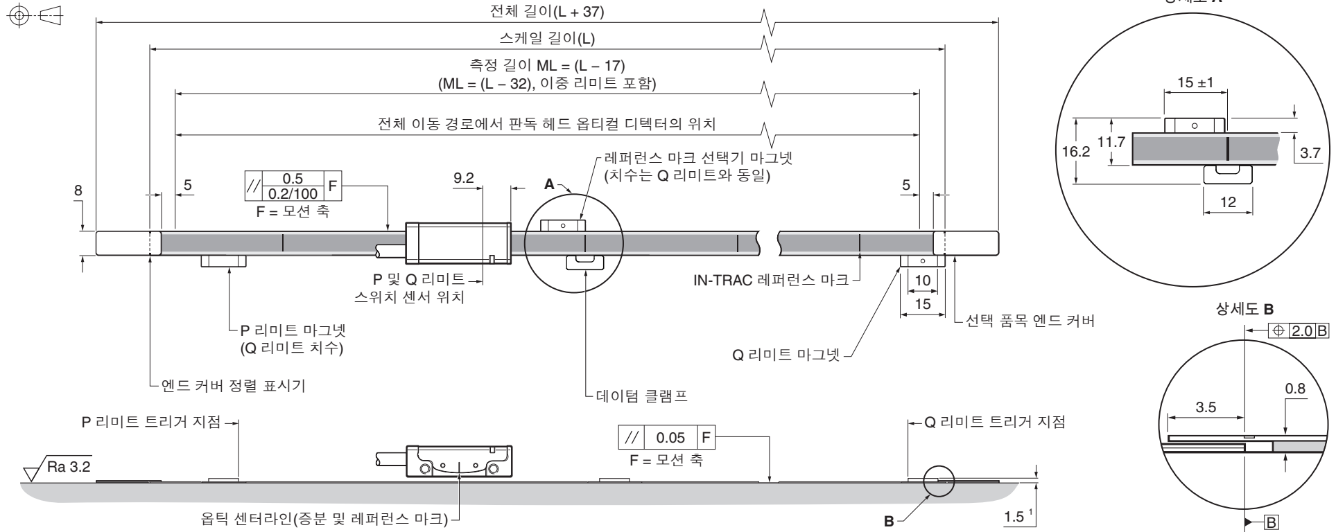
(고객 선택사항) 볼트형 레퍼런스 마크 선택기 및 리미트 마그넷
