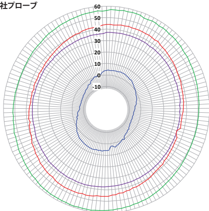
RENGAGE プローブ 単位: \mu\text{m}
