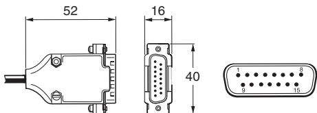
15针D型插头（端子代码D）
