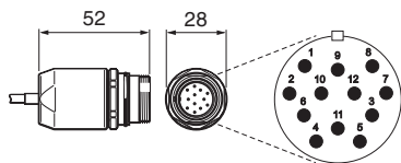
12针圆形连接器（端子代码W）
