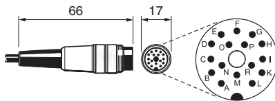
同轴插头（端子代码X）
