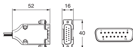
D サブ 15 ピンコネクタ (終端コード D)
