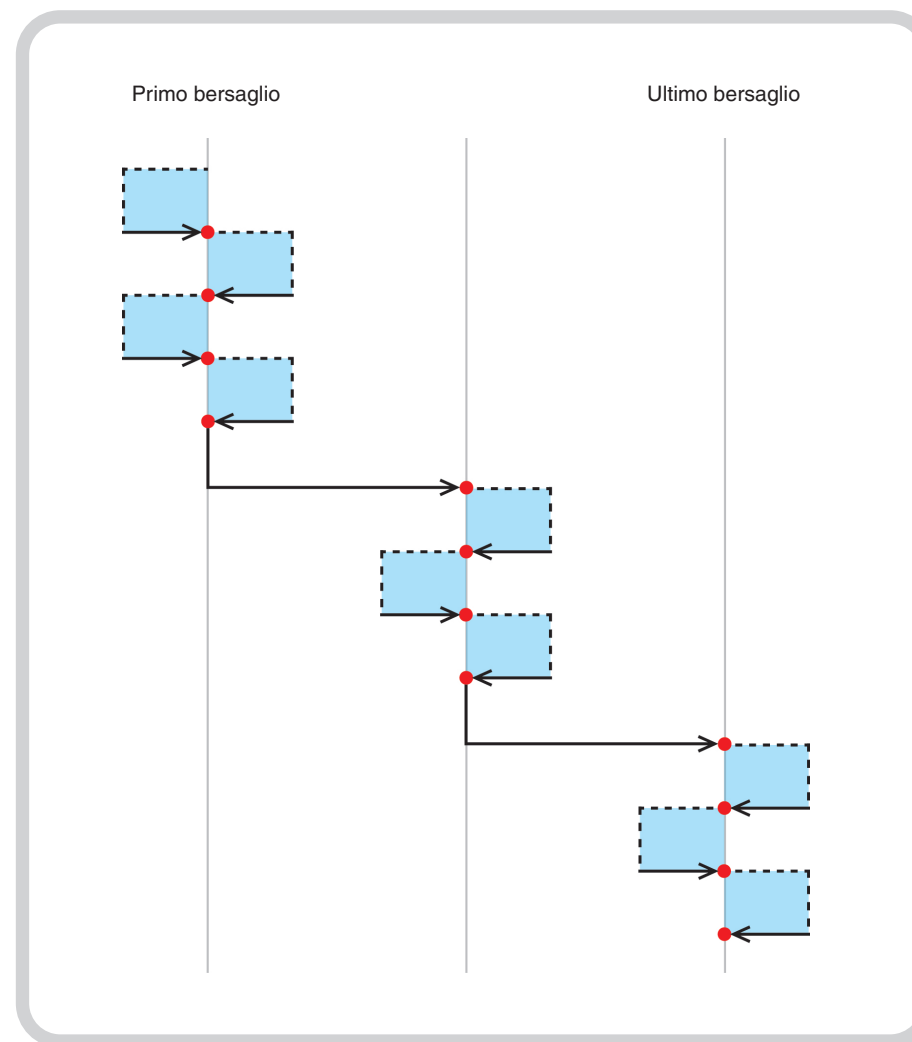
Figura 6 Acquisizione dati a pendolo con due corse bidirezionali.
