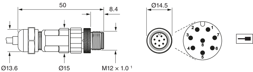
8针M12型插头
