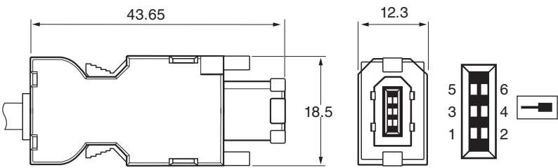
6针Molex型插头
