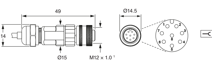
8针M12型插槽
