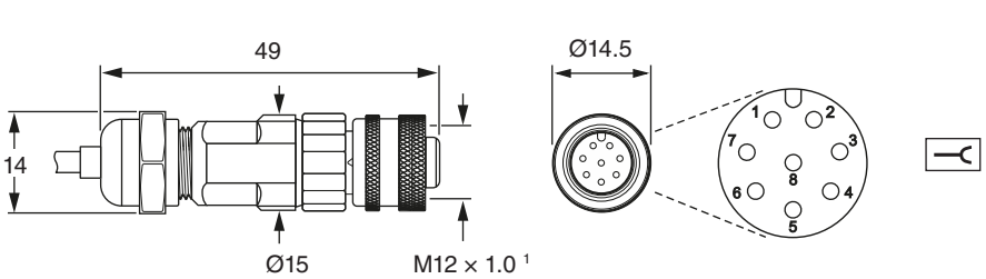
8针M12型插槽
