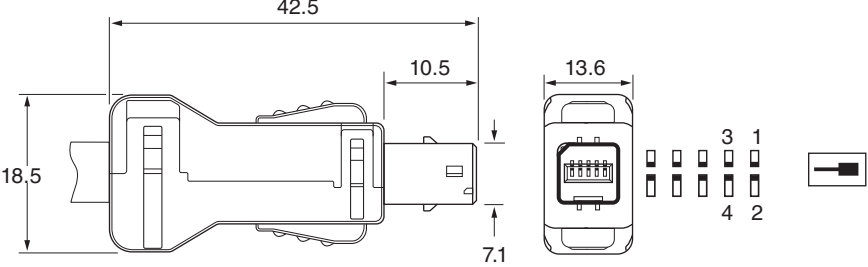
10针JST型插头
