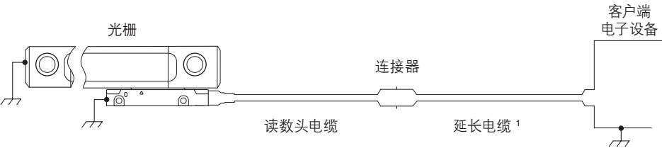
图1 标准布置。
