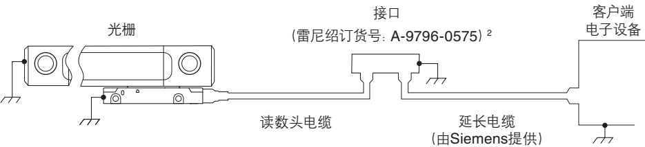
图2 适合Siemens DRIVE-CLiQ型号的布置。
