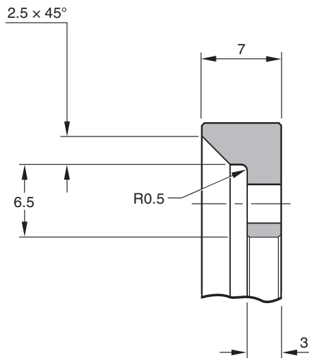
截面A-A
