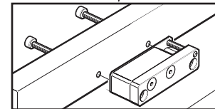
슬림 어플리케이터 A-9402-0060(17페이지 참조)
