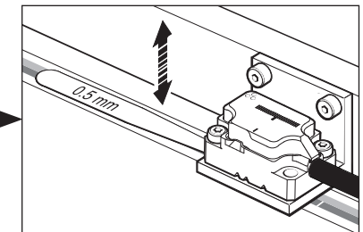
정확한 브래킷 및 틈새 게이지(29페이지 참조)
