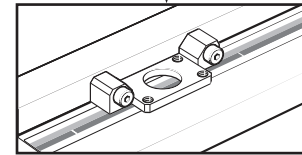
판독 헤드의 데이터 에지가 기계 축에 장착됩니다. 측면 장착 브래킷 A-9401-0103 또는 고객 설계 브래킷과 함께 사용할 수 있습니다.
