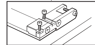
상부 장착 어플리케이터 A-9402-0028 (17페이지 참조)
