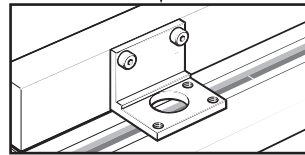
판독 헤드의 데이터 에지가 브래킷 기준면에서 편요각을 제어합니다. 'L' 장착 브래킷 A-9402-0037 또는 고객 설계 브래킷과 함께 사용할 수 있습니다.
