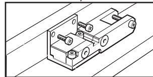
상부 장착 어플리케이터 A-9402-0028(17페이지 참조)
