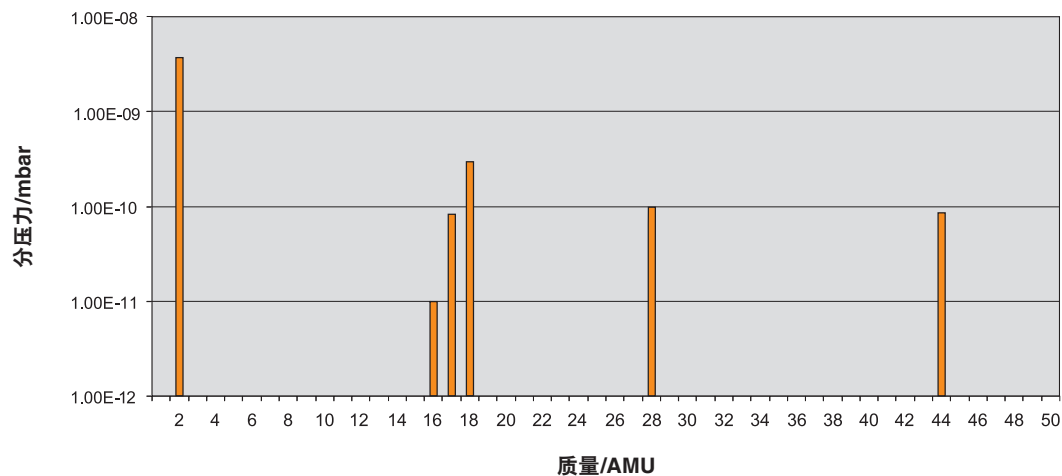
经过烘焙后的RSLA30直线栅尺 (180 mm长, 带2个夹片和1个夹具) (总压力 = 3.0 \times 10^{-10} \text{ mbar} )
