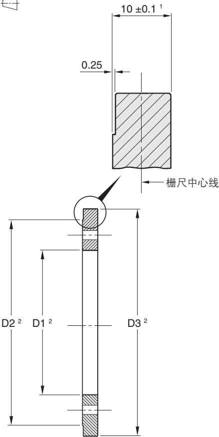
截面A-A
