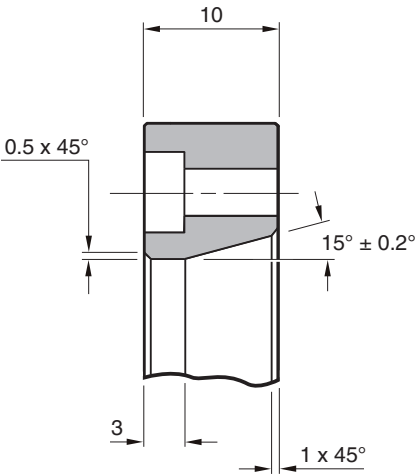
截面A-A
