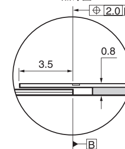
可选螺栓固定式参考零位选择器和限位磁体
