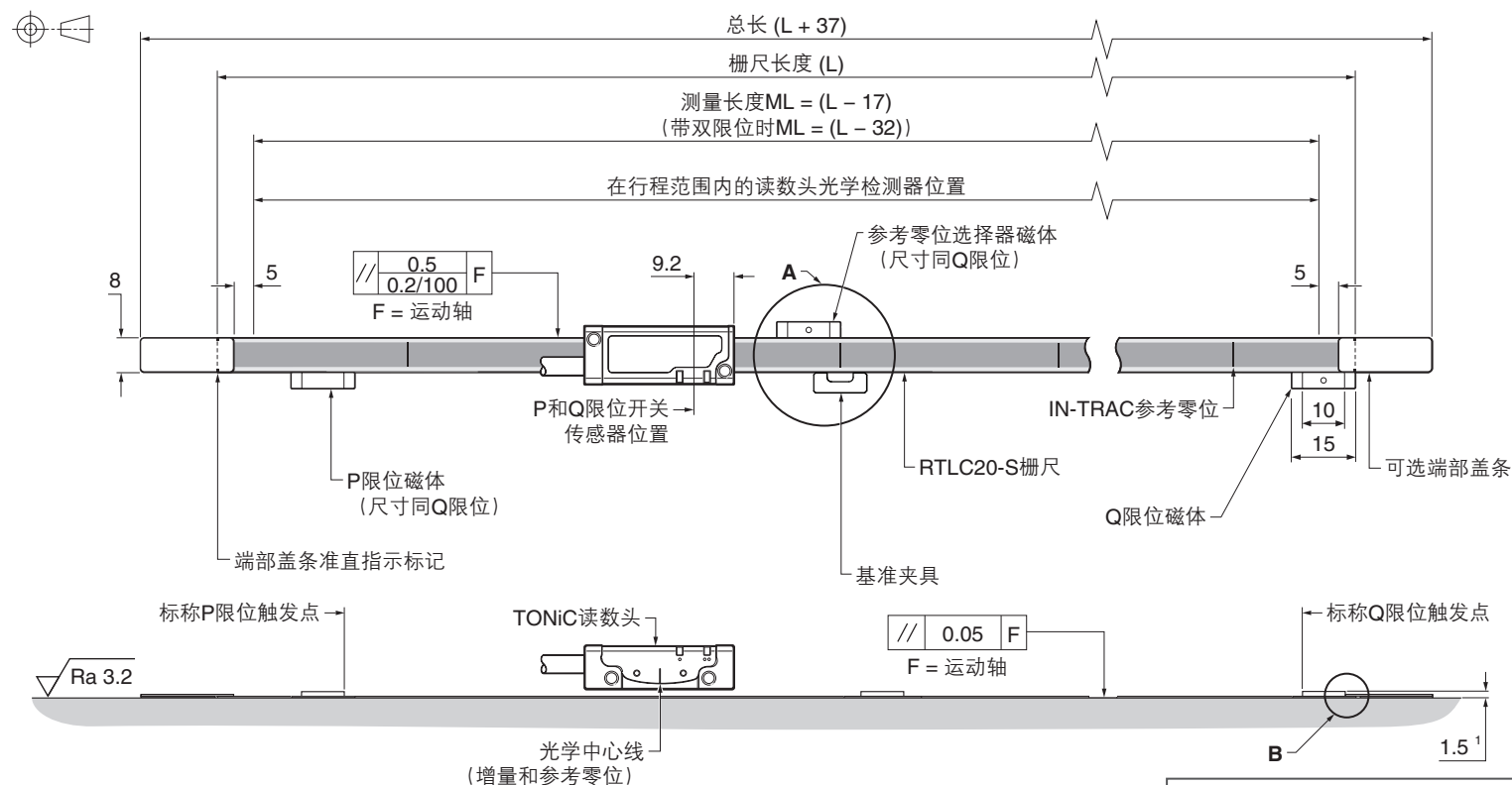
可选螺栓固定式参考零位选择器和限位磁体
