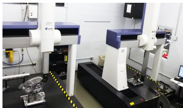
CMM equipaggiata con REVO alla Kawasaki di Maryville
