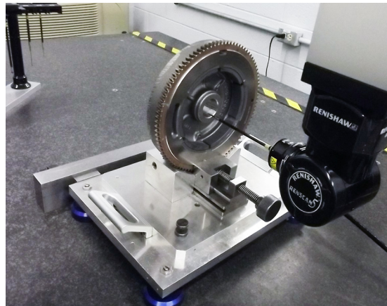
Testa REVO mentre ispeziona il volano di un motore della serie FX
