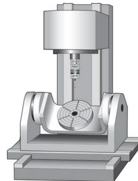
Centres d'usinage 5 axes horizontaux et verticaux avec axes tables rotatifs
