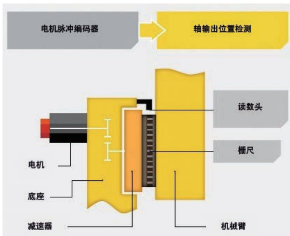
FANUC机器人的定位系统结构。 图片版权归FANUC所有。
