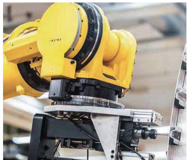
FANUC机械臂的回转轴上配备RESOLUTE绝对式圆光栅。
