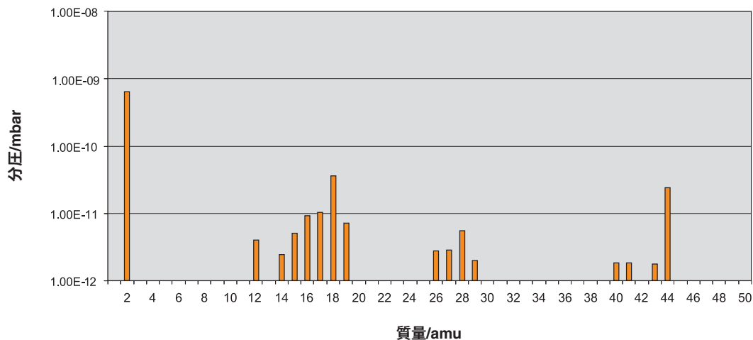
ベーキング後の RSLA30 リニアスケール (スケール長 180mm、クリップ 2 個とクランプ 1 個で固定) (全圧 = 3.0 \times 10^{-10}\text{mbar} )
