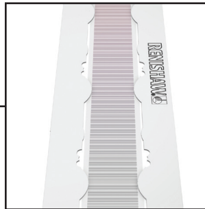
RTLA50 테이프 스케일 및 FASTRACK 캐리어
