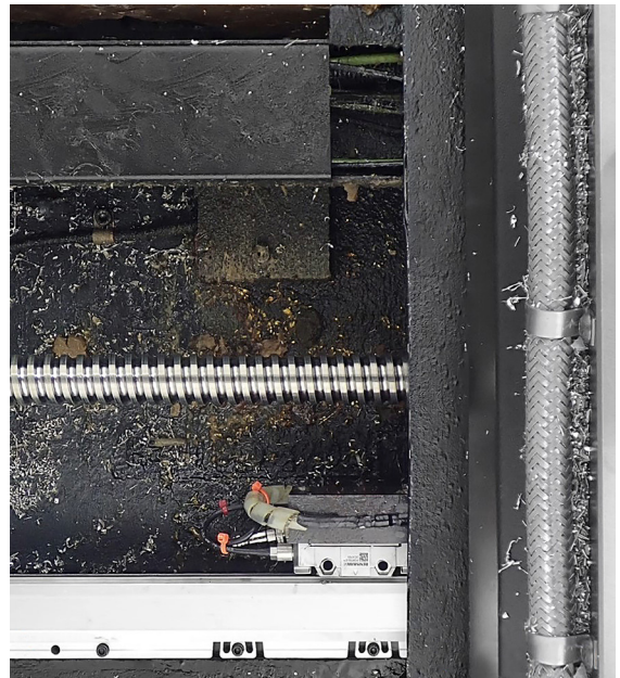
그림 2. 커버로 보호되더라도 리니어 엔코더는 지속적으로 입자·그리스·냉각수에 노출됩니다.
