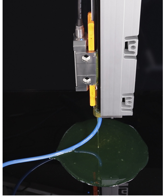
그림 1. 고의로 오일이 유입된 FORTiS 엔코더에서 오일을 배출하는 에어 퍼지
