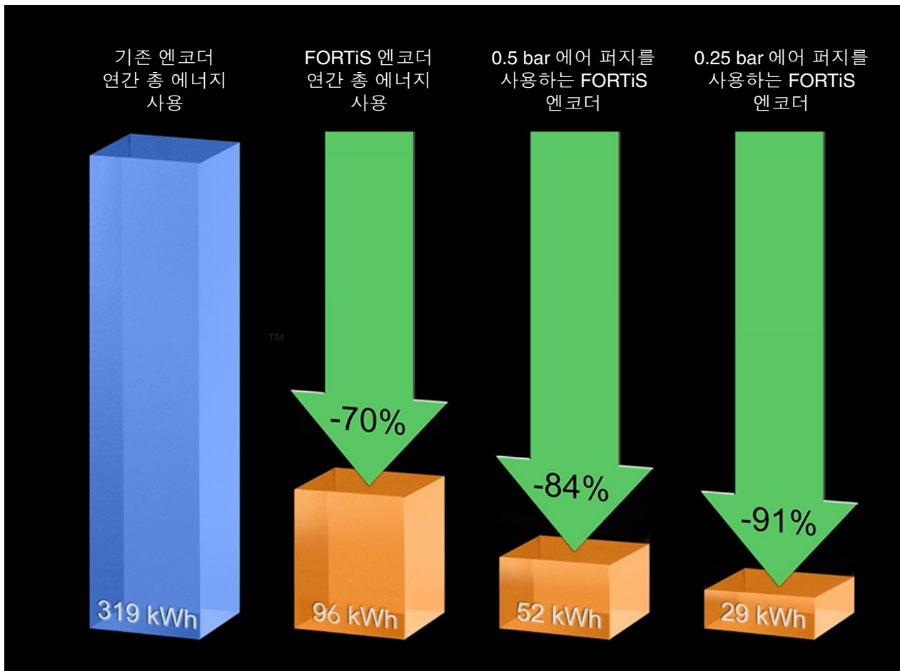
그림 4. 에어 퍼지 사용을 70% 감소시키는DuraSeal™ 립 씬에 “저유량”에어 퍼지 방식을 채택함으로써 더 큰 절감 효과를 얻을 수 있습니다.
